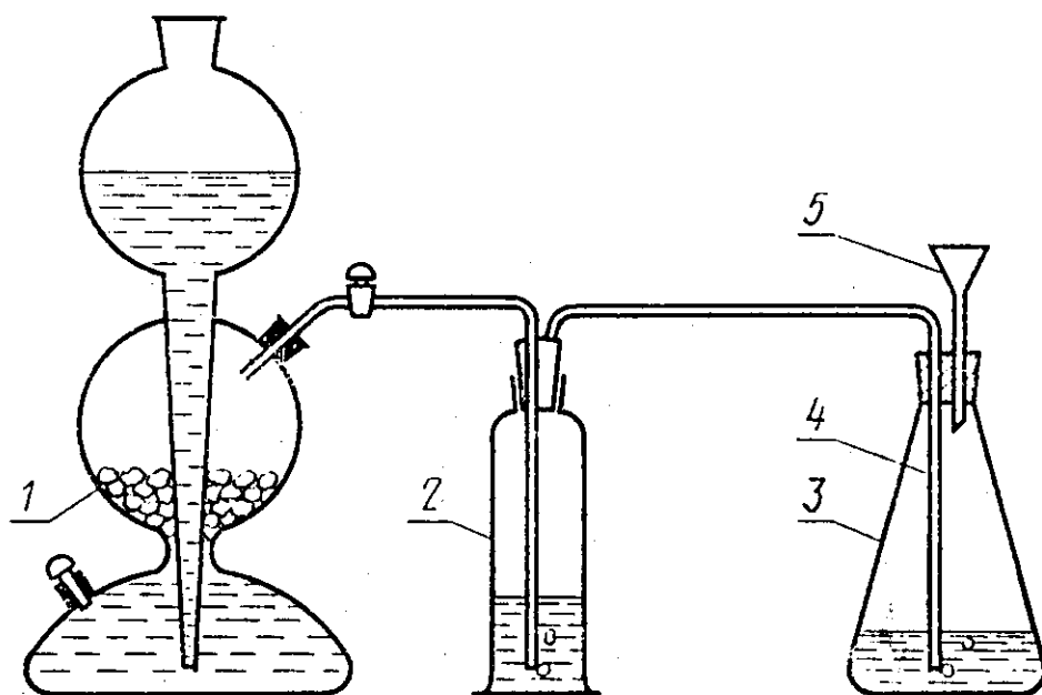
1—аппарат Киппа для получения углекислого газа (заряжают кусками мрамора и соляной кислоты, разбавленной 1:1); 2—склянка Дрекслея, заполненная раствором сернокислой меди; 3—коническая колба вместимостью 500 см 3 ; 4—отводная трубка; 5—воронка
