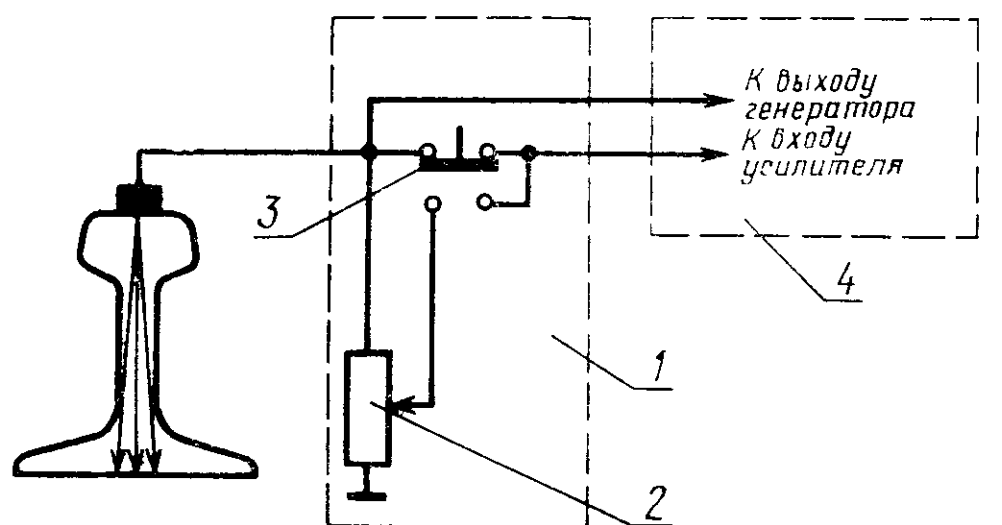
1 — имитатор дефектов; 2 — аттенюатор; 3 — переключатель; 4 — дефектоскоп
