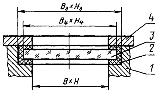
1 — корпус (рама); 2 — герметизирующий материал; 3 — стекло; 4 — рамка
