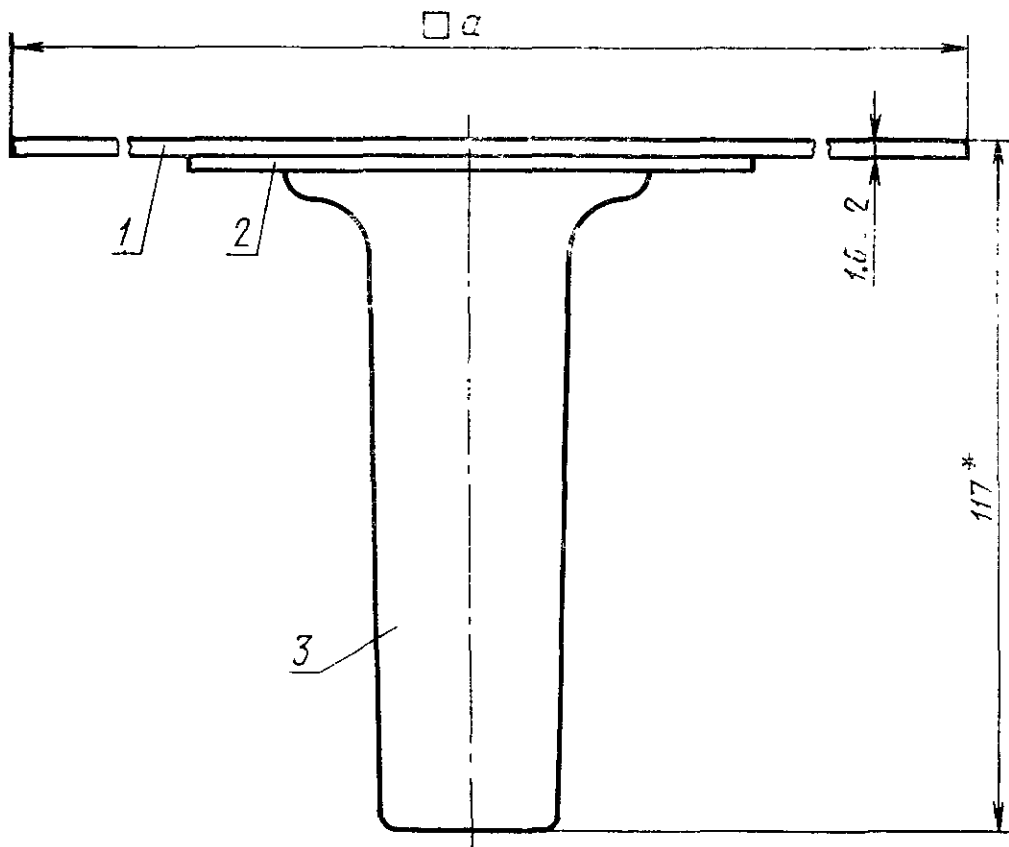
1 — полотно; 2 — фланец; 3 — ручка
