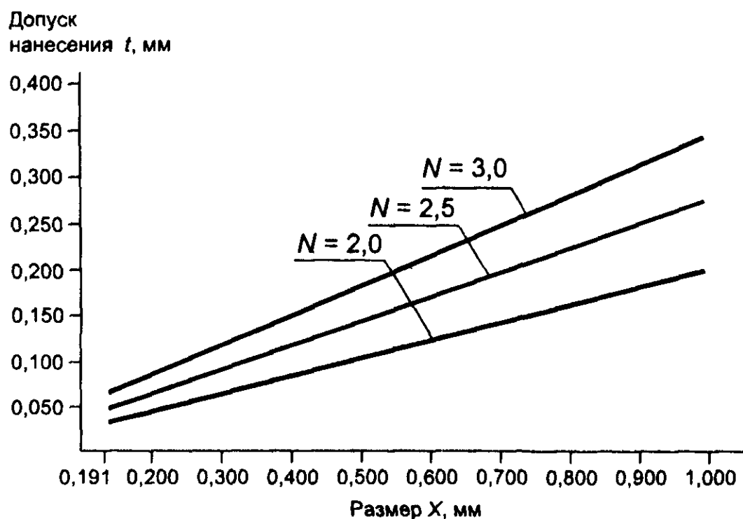
Рисунок 4 — Допуски для “2 из 5 чередующийся”
