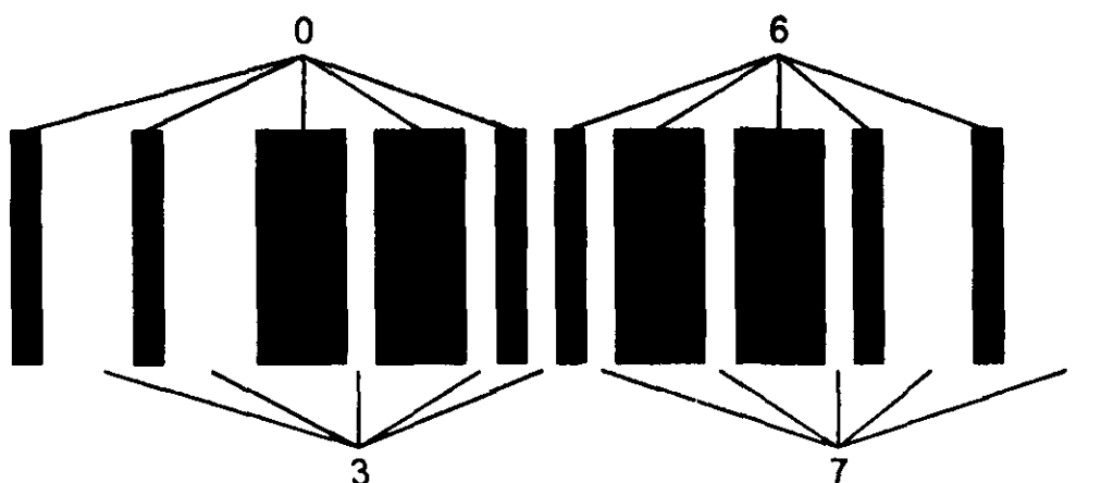
Рисунок 1 — Пары знаков символа “2 из 5 чередующийся”, кодирующие последовательность данных 03 67
