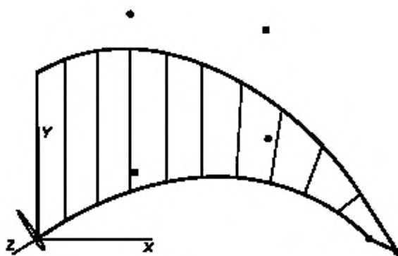
Рисунок E.2 — Графленая поверхность и линия директрисы
