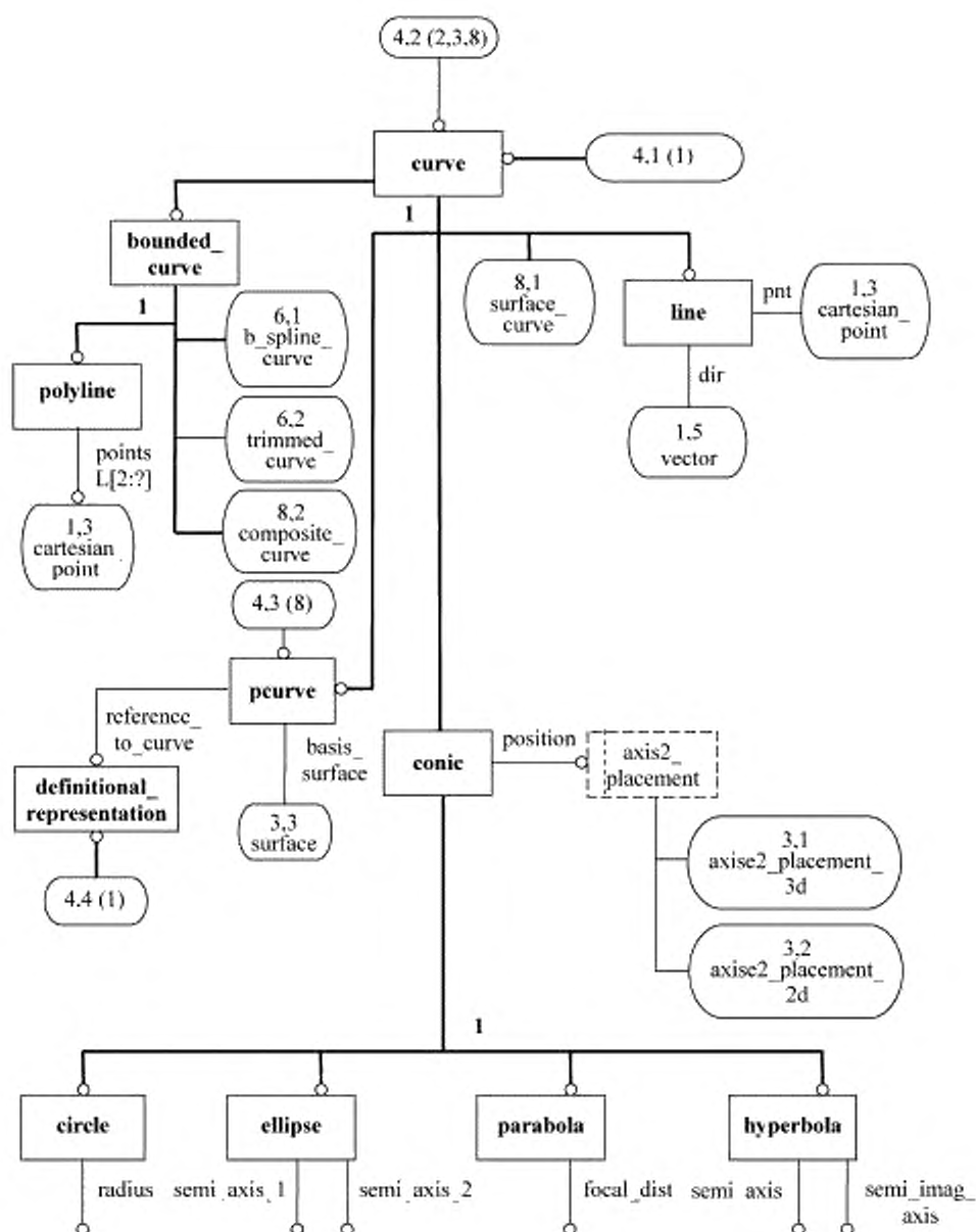
Рисунок D.4 — ПИК alc_curve_swept_solid в формате EXPRESS-G (диаграмма 4 из 9)
