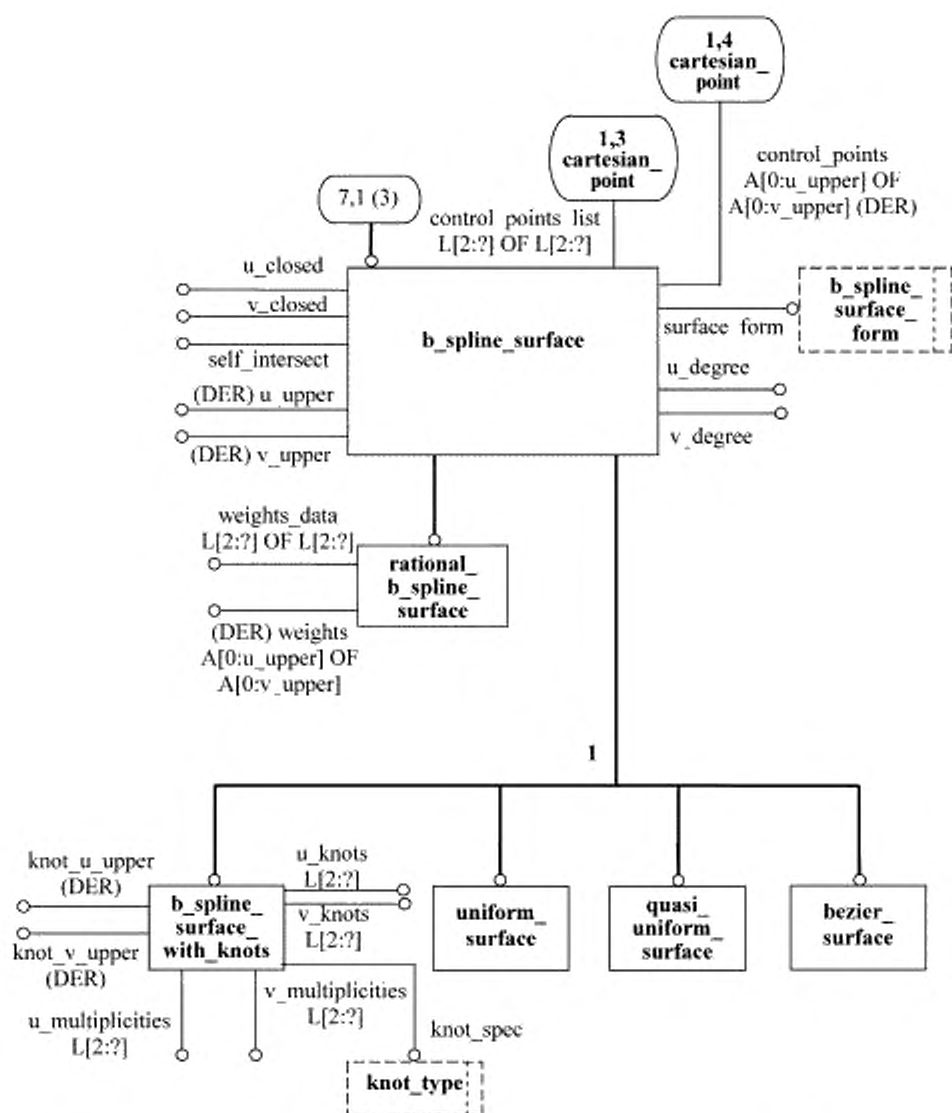
Рисунок D.7 — ПИК alc_curve_swept_solid в формате EXPRESS-G (диаграмма 7 из 9)
