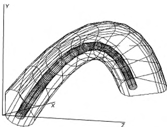
Рисунок E.3 — Представление формы криволинейного изогнутого тела
