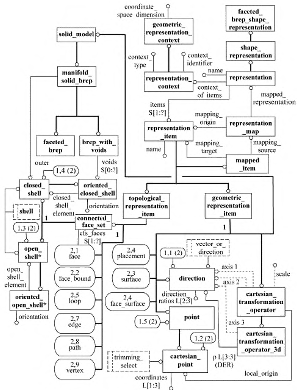
Рисунок D.1 — ПИК alic_faceted_brep в формате EXPRESS-G (диаграмма 1 из 2)
