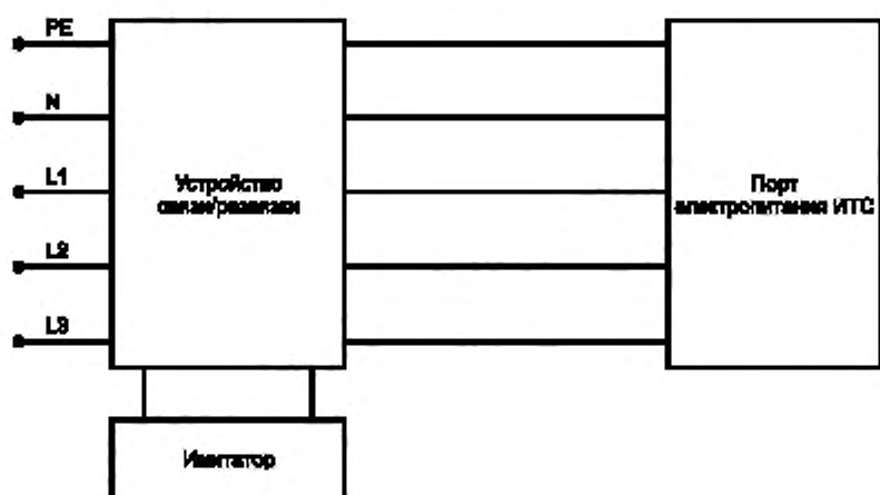
Рисунок Д.2, лист 2
