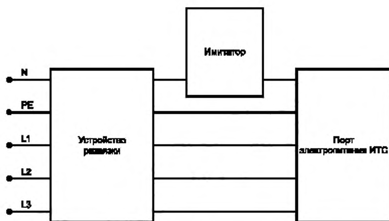
Рисунок Д.1, лист 2
