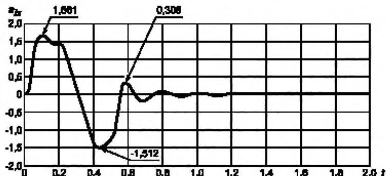
c) Реакция позвоночника в направлении z
