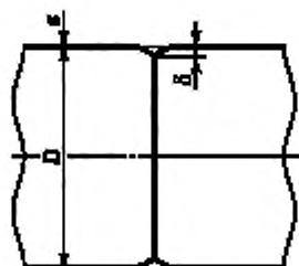
Рисунок А.2 — Увод кромок кольцевого шва
