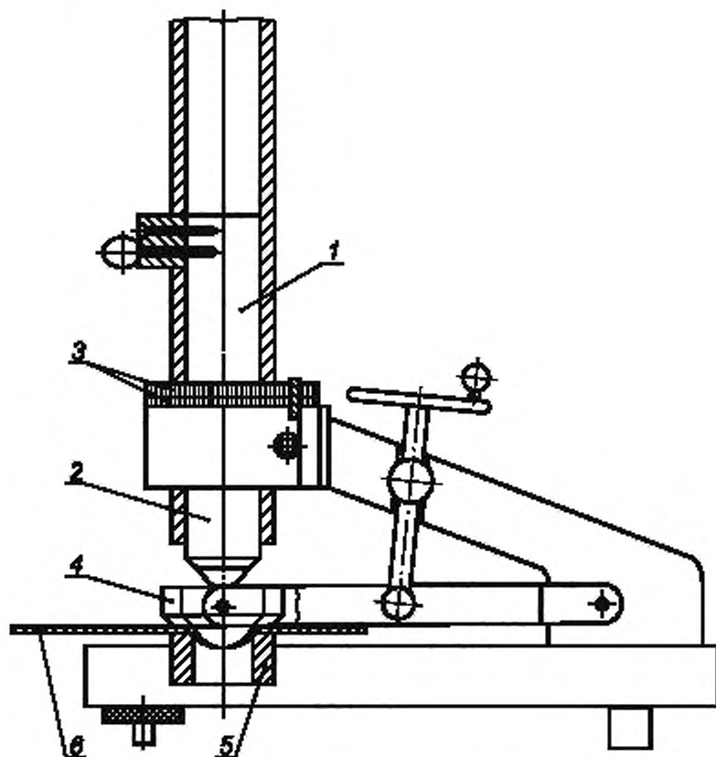
1 — направляющая труба; 2 — падающий груз; 3 — ограничитель; 4 — прижимная муфта; 5 — наковальня; 6 — испытуемая пластинка
