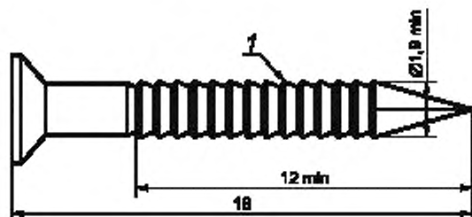
Рисунок 1 — Стандартный каблучный гвоздь
