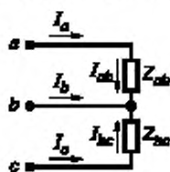
а, б, в — фазы основной вторичной обмотки ТН; I_a, I_b, I_c — фазные токи; I_{ab}, I_{bc} — междофазные токи; Z_{ab}, Z_{bc} — междофазные нагрузки
