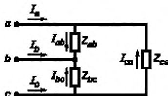
а, б, в — фазы основной вторичной обмотки ТН; I_a, I_b, I_c — фазные токи; I_{ab}, I_{bc}, I_{ca} — междофазные токи; Z_{ab}, Z_{bc}, Z_{ca} — междофазные нагрузки
