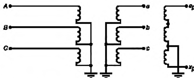
А, В, С — фазы первичной обмотки ТН; а, б, в — фазы основной вторичной обмотки ТН; a_D, b_D, c_D — фазы дополнительной вторичной обмотки ТН
