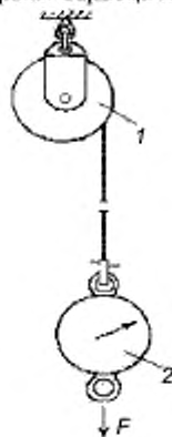
1 — УКСПа; 2 — динамометр
