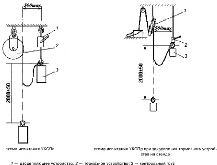
Рисунок 5 — Схемы испытания УКСП на динамическую прочность
