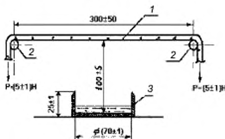
1 — образец каната (ленты); 2 — опоры; 3 — емкость для горючего
