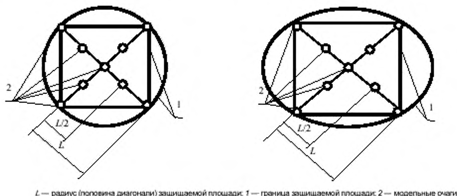
L — радиус (половина диагонали) защищаемой площади; 1 — граница защищаемой площади; 2 — модельные очаги
