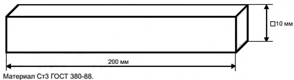
Рисунок А.1 — Стержень для проведения испытания по 8.11
