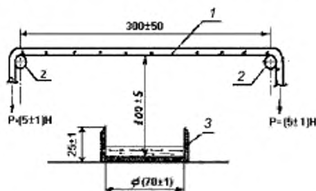
1 — образец веревки; 2 — опоры; 3 — емкость для горючего
