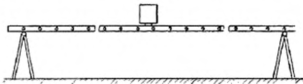
Рисунок 1 — Схема установки лестницы на опоры
