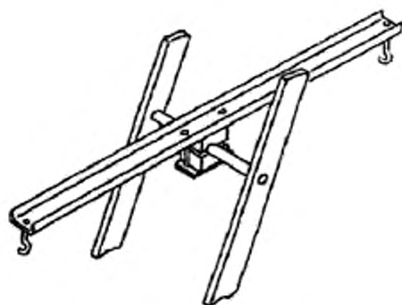
Рисунок 7 — Приспособление для испытания ступеньки на кручение
