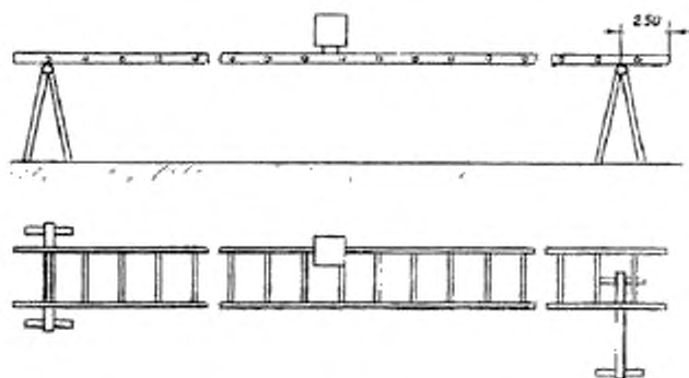
Рисунок 3 — Схема установки или подвески контрольного груза
