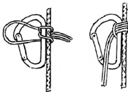
Рисунок 11 — Карабинный узел
