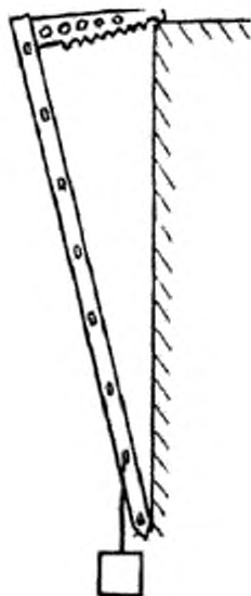
Рисунок 15 — Схема испытания крюка штурмовой лестницы на прочность
