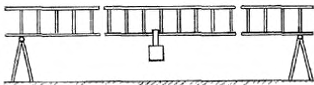
Рисунок 2 — Схема подвески контрольного груза
