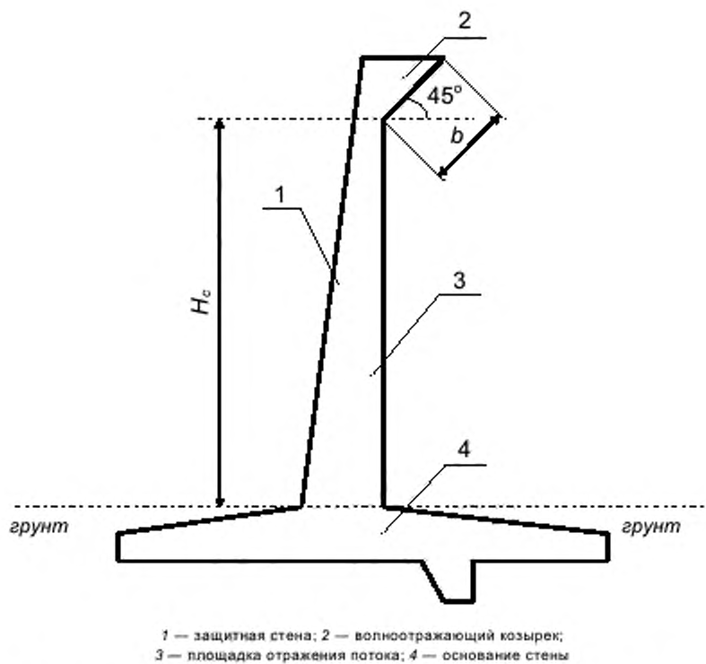
Рисунок А.1 — Принципиальная схема ограждающей стены с волноотражающим козырьком
