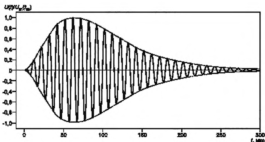
Рисунок 2 — Типичная форма радиоимпульса с экспоненциально-степенной огибающей.
