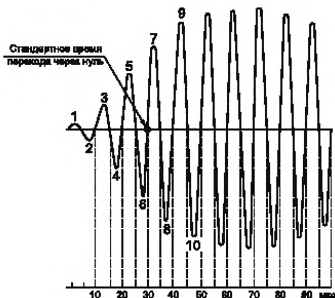
Рисунок 3 — Моменты времени переходов колебаний ВЧ через нуль и обозначения полувольт
