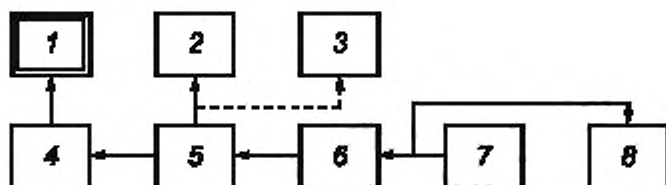
1 — испытуемое оборудование; 2 — анализатор спектра; 3 — измеритель модуляции (девиометр); 4 — аттенуатор (при необходимости); 5 — делитель мощности; 6 — высокочастотный генератор сигналов; 7 — низкочастотный генератор сигналов; 8 — частотомер
