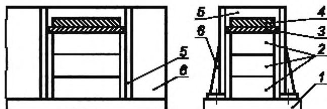
1 — стол вибростенда; 2 — испытуемые образцы; 3, 4 — плита, создающая нагрузку, 5, 6 — ограждение, ограничивающее перемещение образцов и плит
