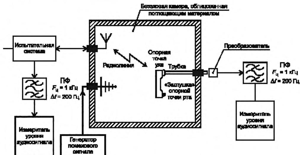
Рисунок 2 — Схема прохождения сигнала при испытаниях радиооборудования
