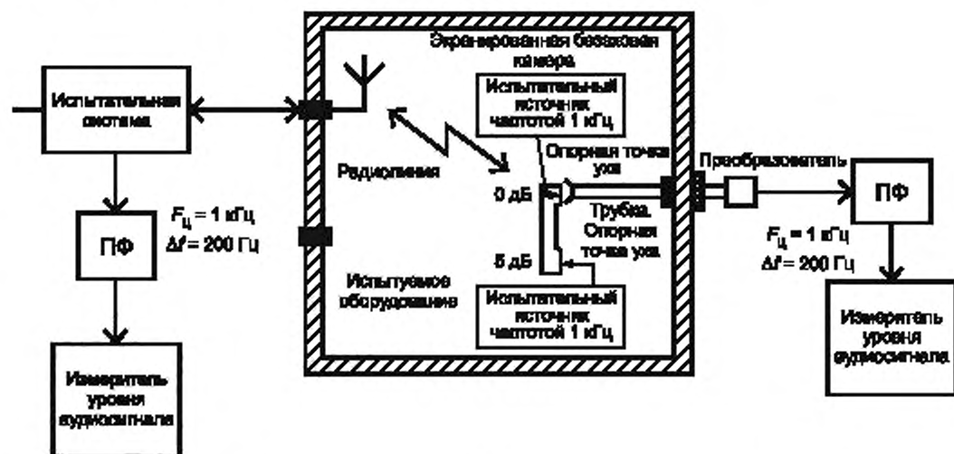
ПФ — полосовой фильтр; F_{ц} — центральная частота полосы пропускания полосового фильтра; \Delta f — полоса пропускания фильтра
