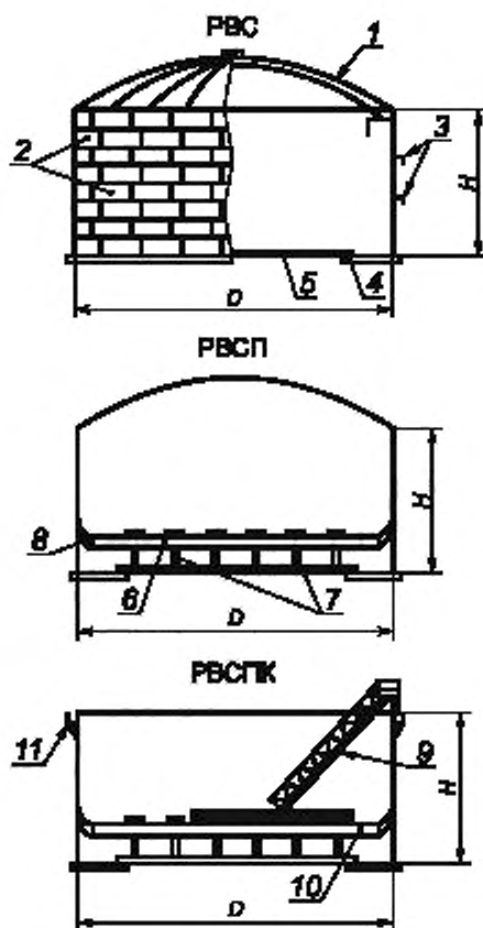
1 — каркас крыши; 2 — пояса стенки; 3 — промежуточные кольца жесткости; 4 — кольцо окраек; 5 — центральная часть днища; 6 — лонтон; 7 — опорные стойки; 8 — уплотняющий затвор; 9 — катуная лестница; 10 — плавающая крыша; 11 — верхнее кольцо жесткости (площадка обслуживания)
