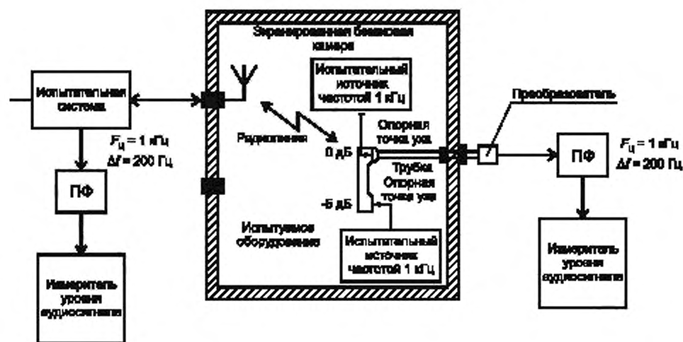
Рисунок 1 — Схема прохождения сигнала при испытаниях
