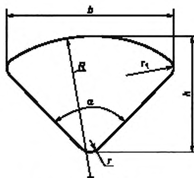
Рисунок А.2 — Конструкция секторных однопроволочных алюминиевых жил
