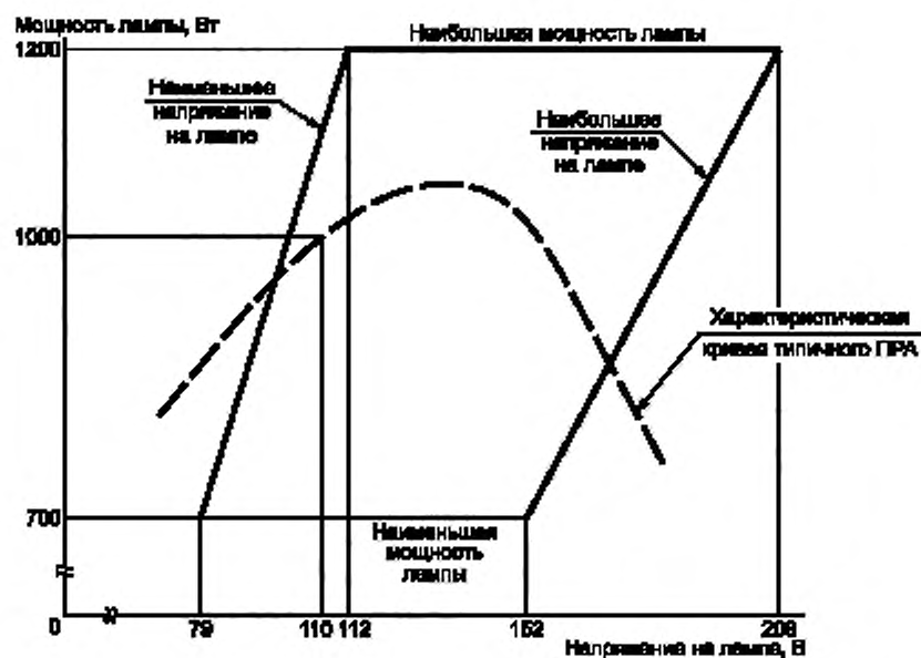
Рисунок Н.8 — Предельные рабочие характеристики лампы номинальной мощностью 1000 Вт с эллипсоидной с диффузным покрытием колбой
