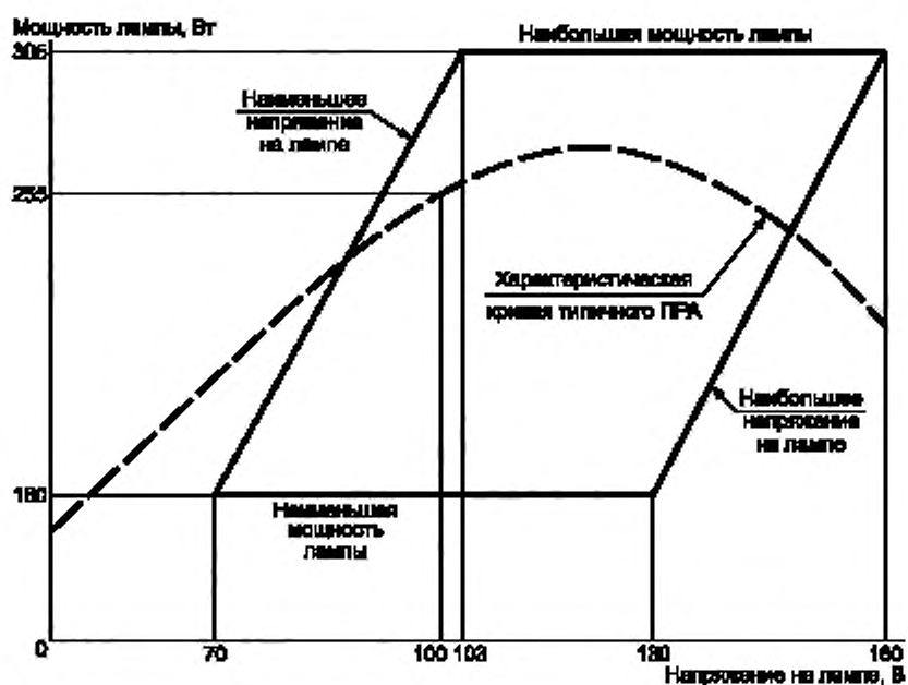
Рисунок Н.14 — Предельные рабочие характеристики лампы номинальной мощностью 250 Вт с повышенным напряжением зажигания, с прозрачной трубчатой или эллипсоидной с диффузным покрытием колбой
