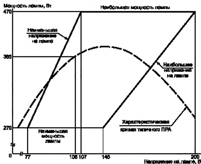
Рисунок Н.13 — Предельные рабочие характеристики лампы улучшенной цветности номинальной мощностью 400 Вт с эллипсоидной с диффузным покрытием колбой
