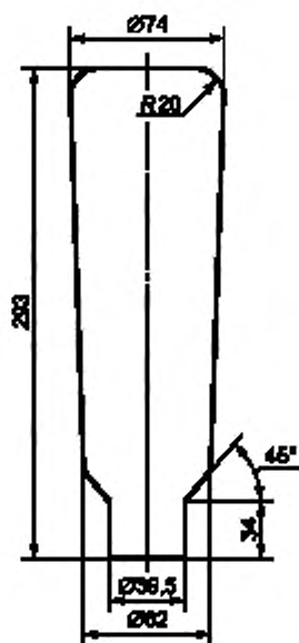
Рисунок G.3 — Трубчатая лампа мощностью 400 Вт
