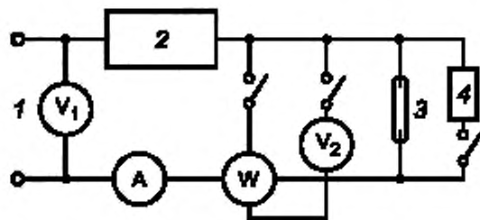
1 — источник питания; 2 — ДОО; 3 — лампа; 4 — ЗУ (тип 1)
