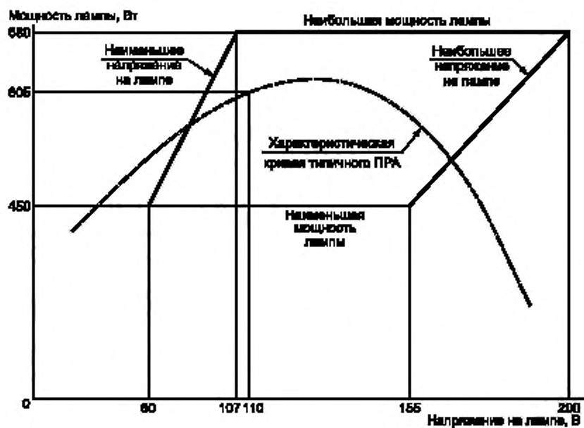
Рисунок Н.17 — Предельные рабочие характеристики лампы номинальной мощностью 600 Вт с трубчатой прозрачной колбой
