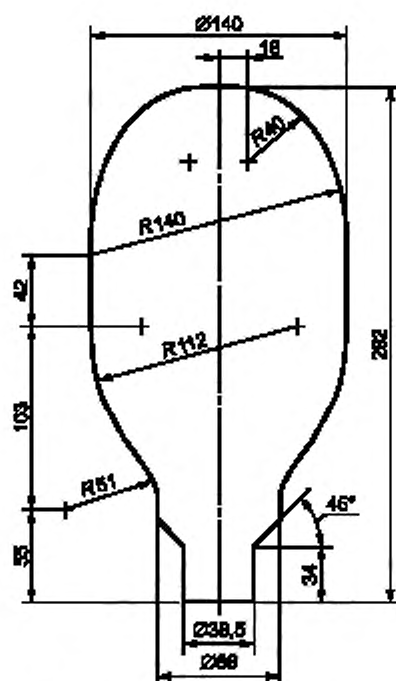
Рисунок G.4 — Эллипсоидная лампа мощностью 400 Вт
