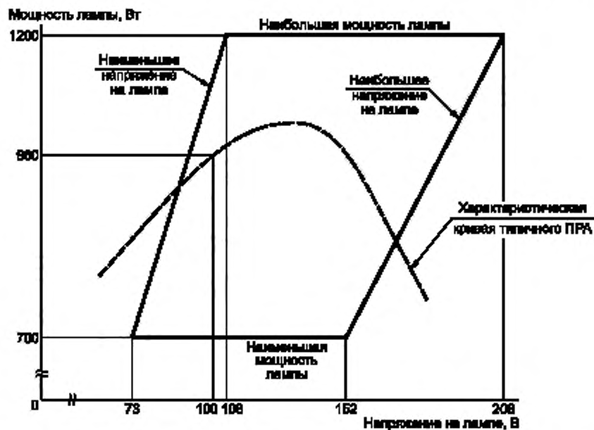
Рисунок Н.7 — Предельные рабочие характеристики лампы номинальной мощностью 1000 Вт с прозрачной трубчатой колбой
