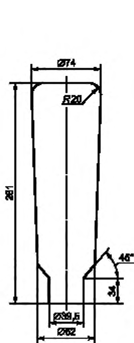
Рисунок G.1 — Трубчатая лампа мощностью 250 Вт
