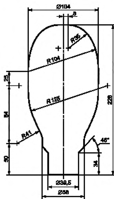
Рисунок G.2 — Эллипсоидная лампа мощностью 250 Вт
