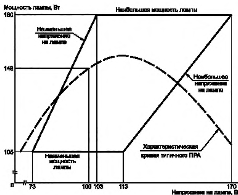
Рисунок Н.10 — Предельные рабочие характеристики лампы улучшенной цветности номинальной мощностью 150 Вт с прозрачной трубчатой или эллипсоидной с диффузным покрытием колбой
