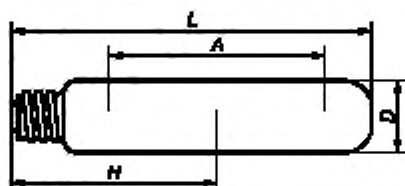
Рисунок В.1 — Лампа с трубчатой колбой
