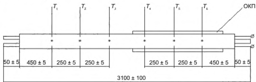
Рис. 1 — Размещение термоэлектрических преобразователей
