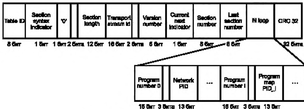
Рисунок А.4 — Диаграмма полей секций таблицы PAT
