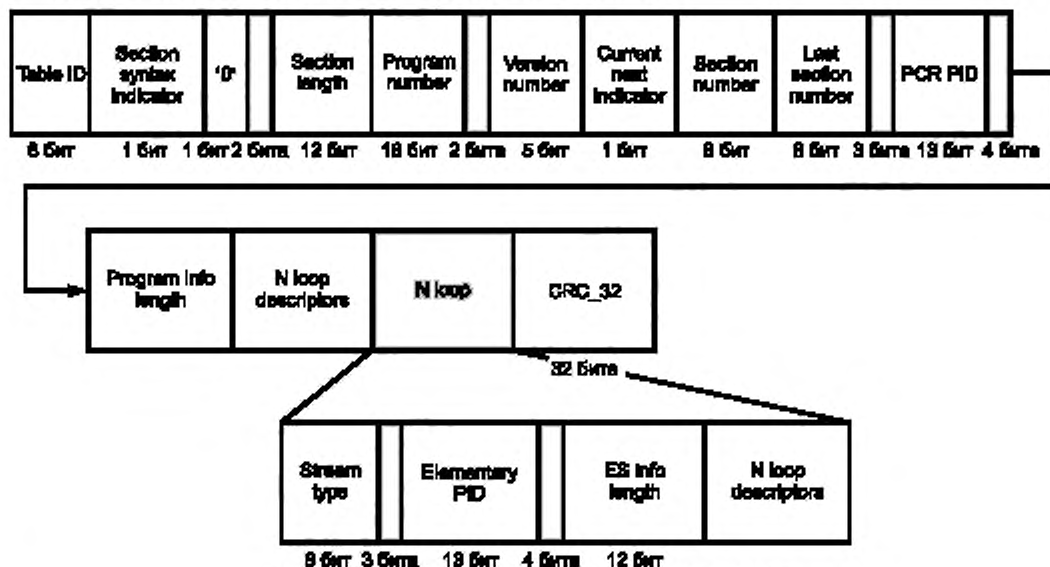
Рисунок А.6 — Диаграмма полей секций таблицы PMT
