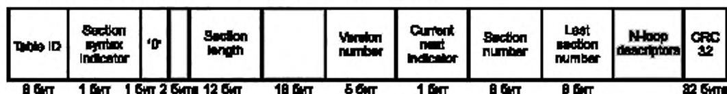
Рисунок А.5 — Диаграмма полей секции таблицы CAT
