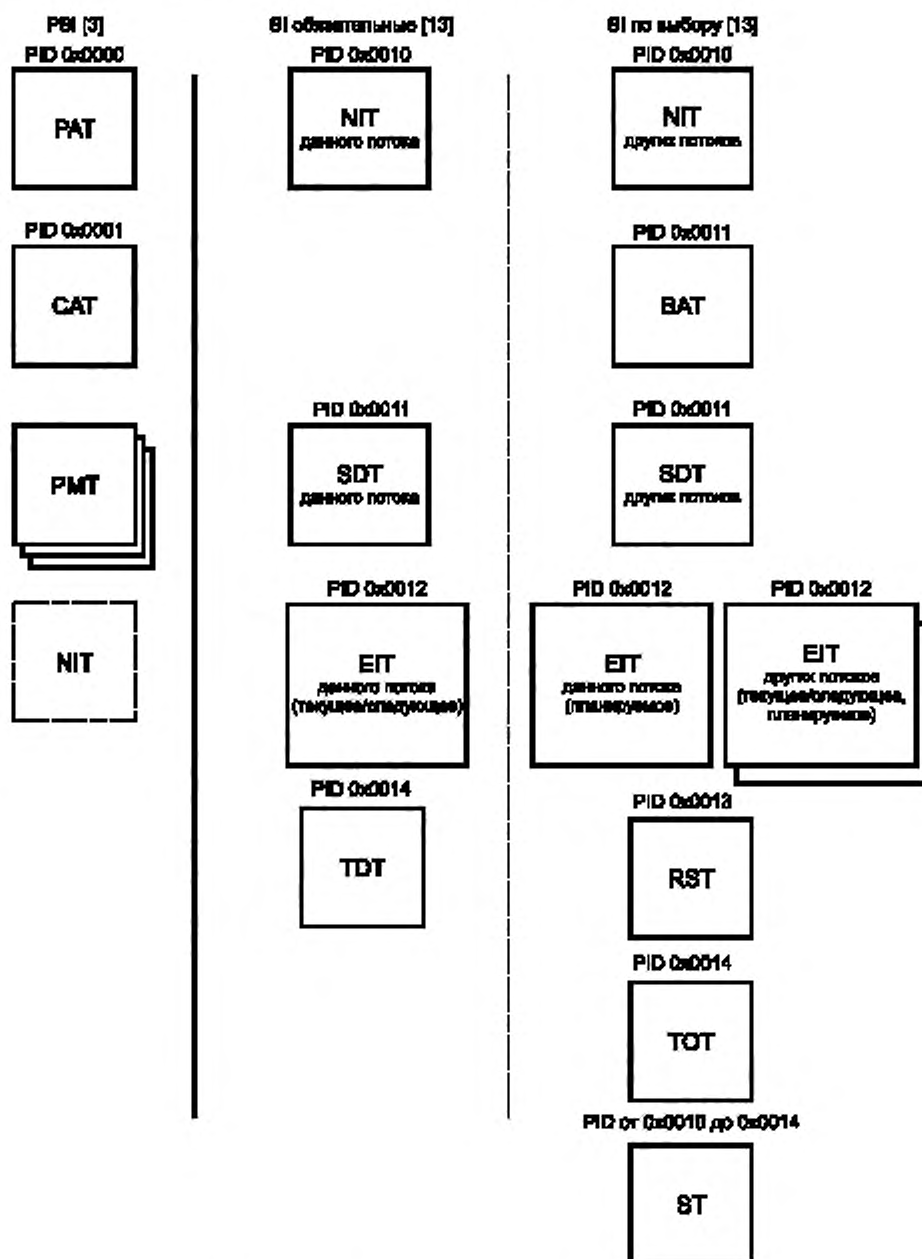
Рисунок А.3 — Полная совокупность таблиц PSI, SI
