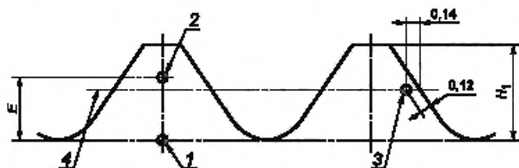
Рисунок 2 — Измерение твердости в испытании на обезуглероживание
