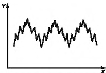
Рисунок 4 — Частотные составляющие сложного сигнала
