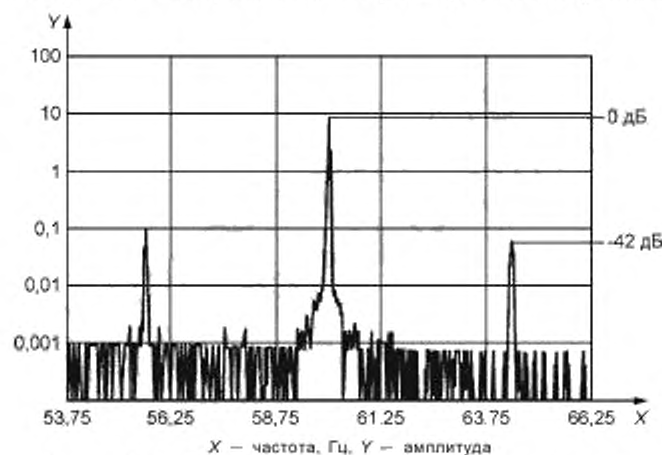
Рисунок 18 — Спектр вибрации неисправного электродвигателя
