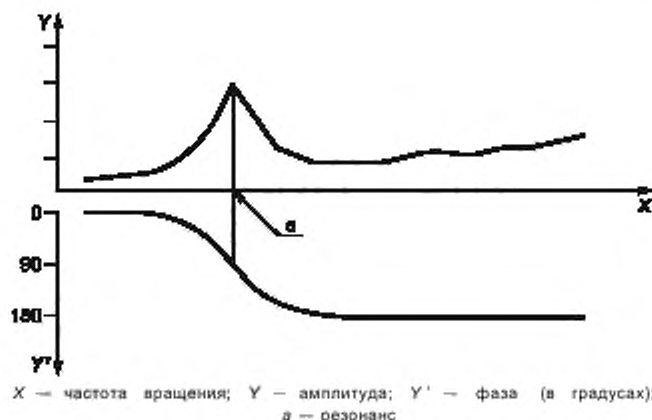
Рисунок 21 — Диаграмма Бode
