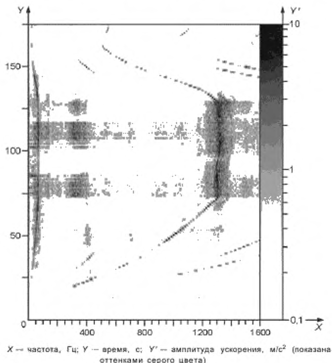
Рисунок 25 — Двумерная спектрограмма
