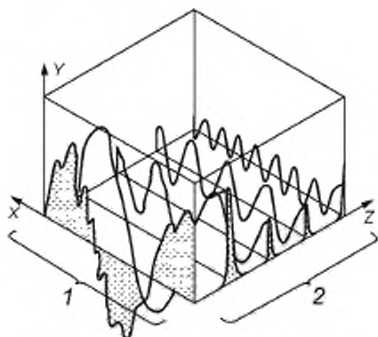
Рисунок 1 — Представление сигнала во временной и частотной областях
