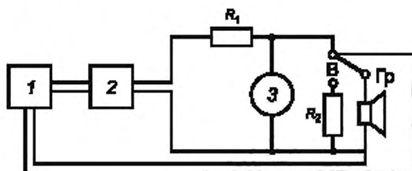
1 — установка для автоматической записи частотной характеристики, 2 — усилитель мощности, 3 — вольтметр (п. 5.4.1), R1 и R2 — активные сопротивления; Гр — громкоговоритель; B — переключатель
