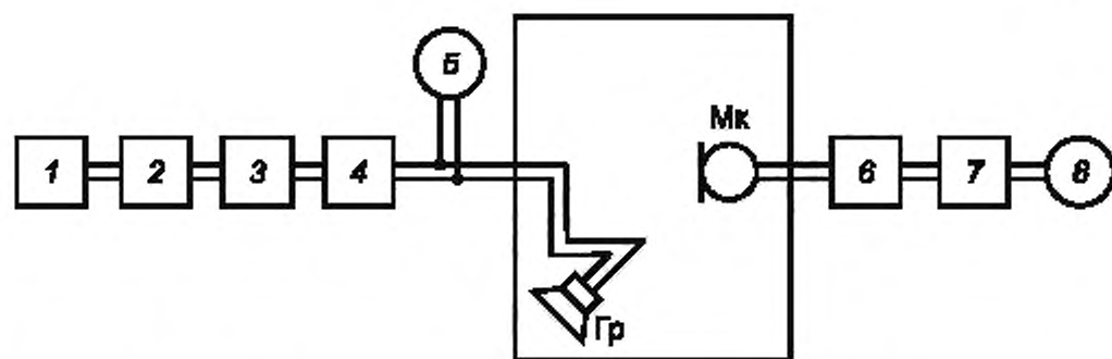
1 — генератор белого шума, 2 — фильтр розового шума, 3 — фильтр полосовой 1/3-октавный; 4 — усилитель мощности; 5, 8 — вольтметры (5.4.2); 6 — усилитель микрофонный; 7 — фильтр полосовой 1/3-октавный с частотой пропускания, кратной частоте пропускания фильтра 3; Мк — измерительный микрофон; Гр — громкоговоритель
