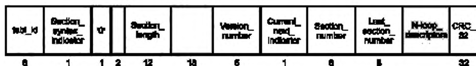
Рисунок A.4 — Структура полей секции таблицы CAT
