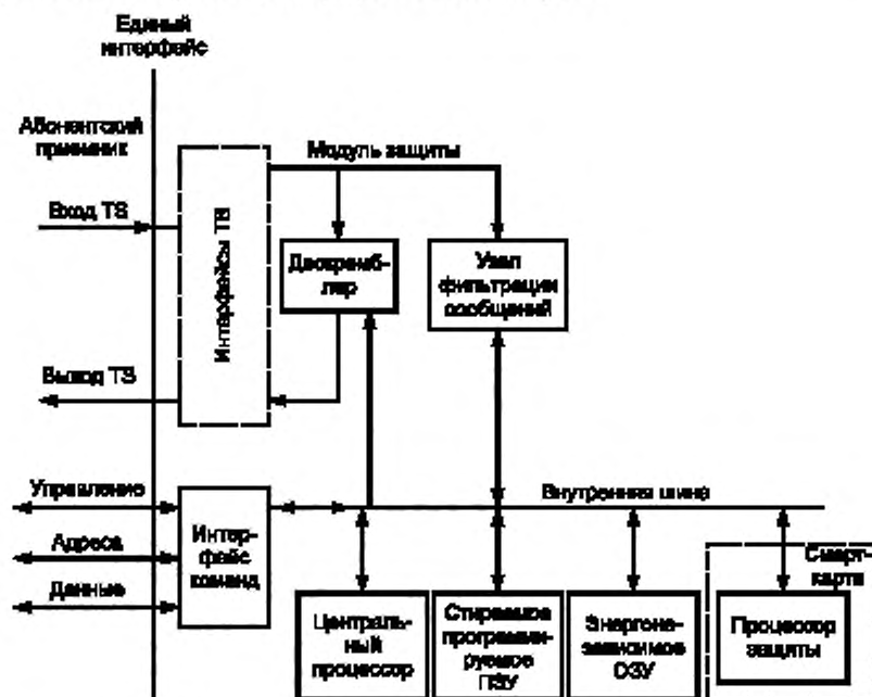
Рисунок 7 — Структурная схема модуля защиты
