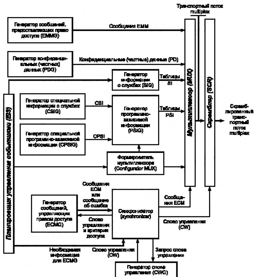
Рисунок 5 — Структурная схема передающей части оборудования СОД Multicrypt
