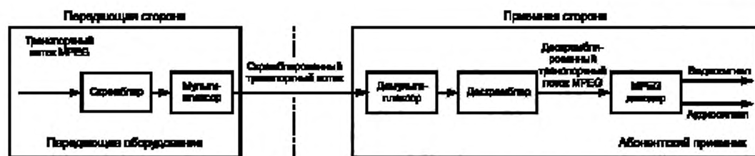
Рисунок 1 — Структурная схема одноуровневой СОД
