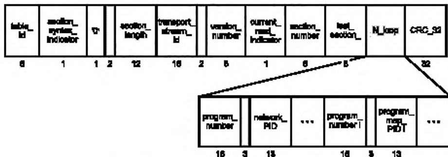
Рисунок A.3 — Структура полей секции таблицы PAT
