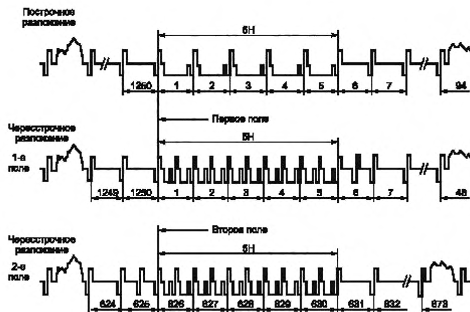
Рисунок 4 — Структура синхросигнала на интервале гашения поля
