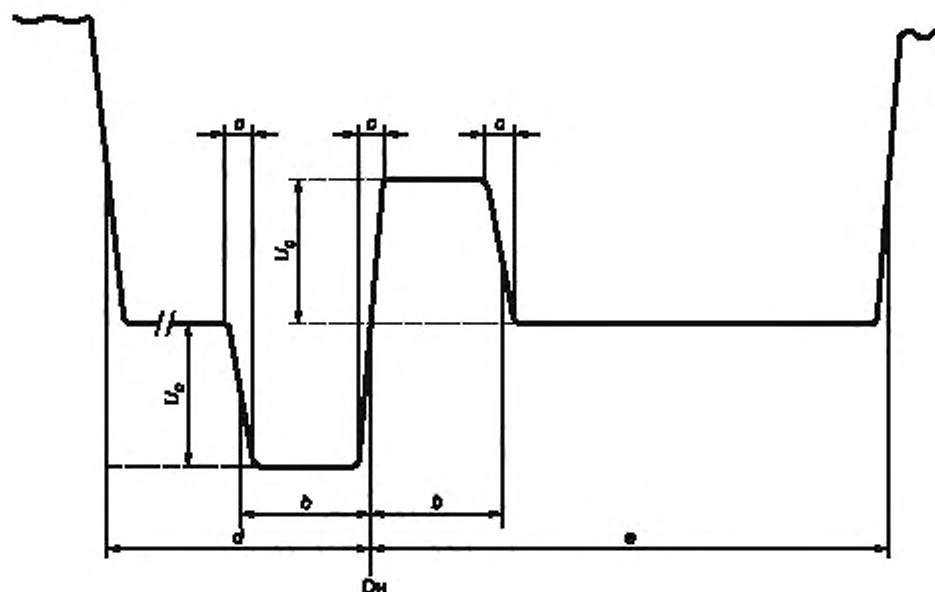
Рисунок 3 — Структура сигнала синхронизации на интервале гашения строки
