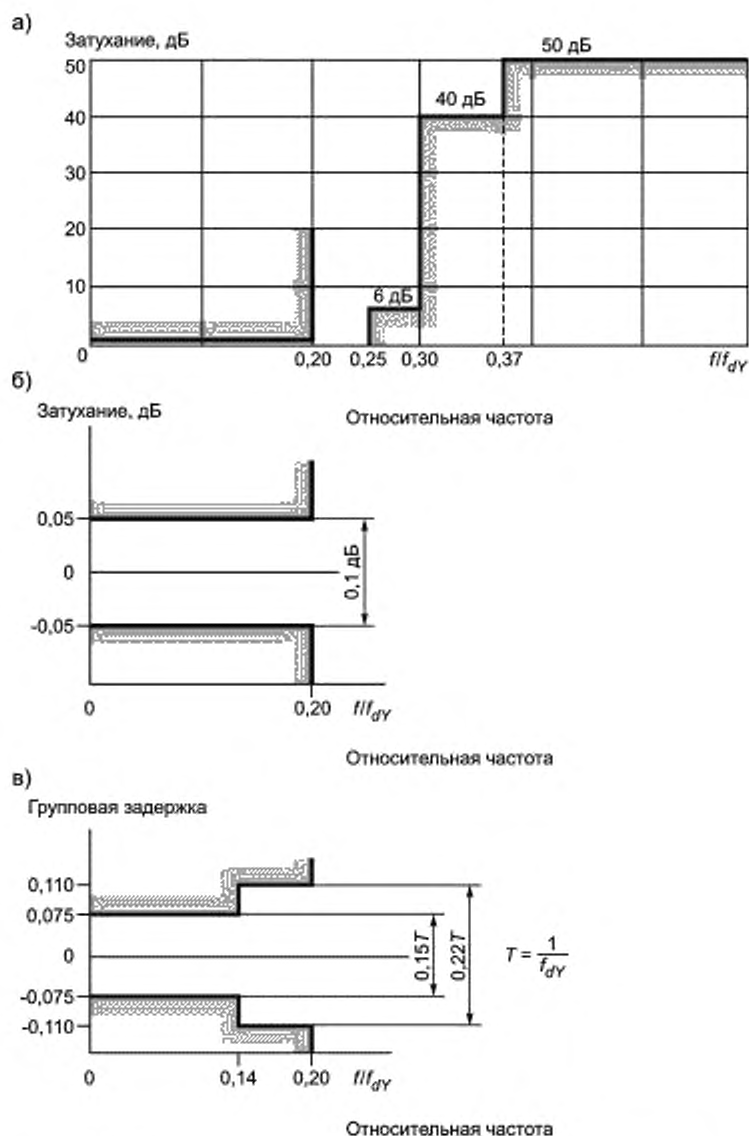
Рисунок 6 — Характеристики фильтров низких частот для сигналов E_{CR}^L и E_{CB}^L
