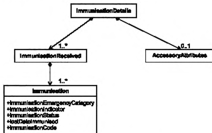
Рисунок 4 — Структура класса информационных объектов «ImmunizationDetails»
