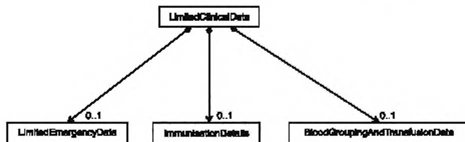
Рисунок 2 — Структура класса «LimitedClinicalData»
