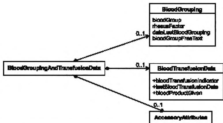
Рисунок 5 — Структура класса информационных объектов «BloodGroupingAndTransfusionData»
