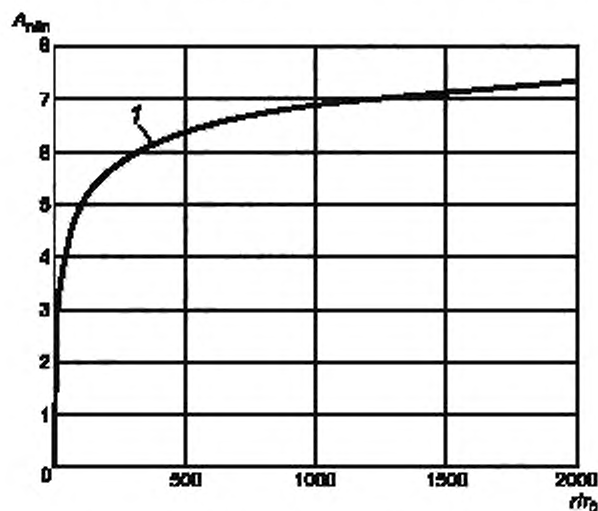
1 — M = 1,3 ; r_0 = 1 м; k = 0,8/340 м -1 ; A_{нлн} — нелинейное затухание, дБА; r — расстояние от точки источника до точки наблюдения, м
