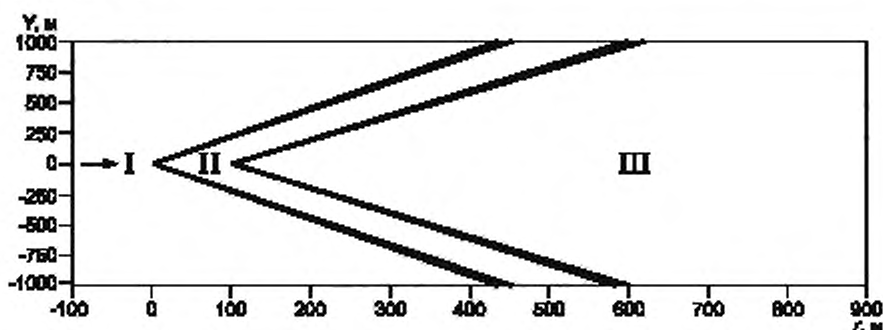
Рисунок А.1 — Границы области II
