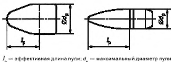
Рисунок 1 — Эффeктивная длина пули
