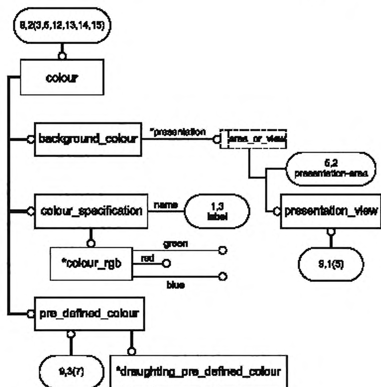
Рисунок С.9 — ПИК aic_mechanical_design_shaded_presentation в формате EXPRESS-G (диаграмма 9 из 16)
