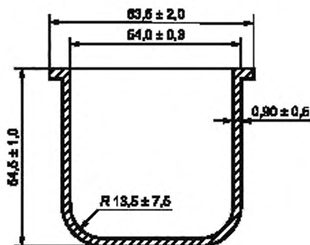
Рисунок A1.1 — Испытательный тигель
