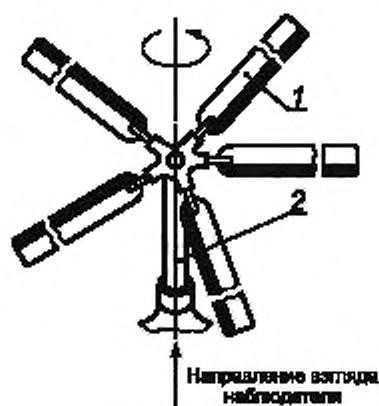
1 — винт, 2 — вал
