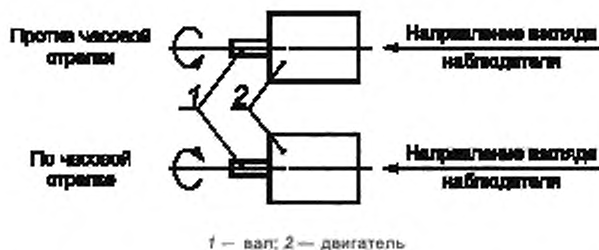
Рисунок 8 — Пример определения направления вращения основного вала ПД
