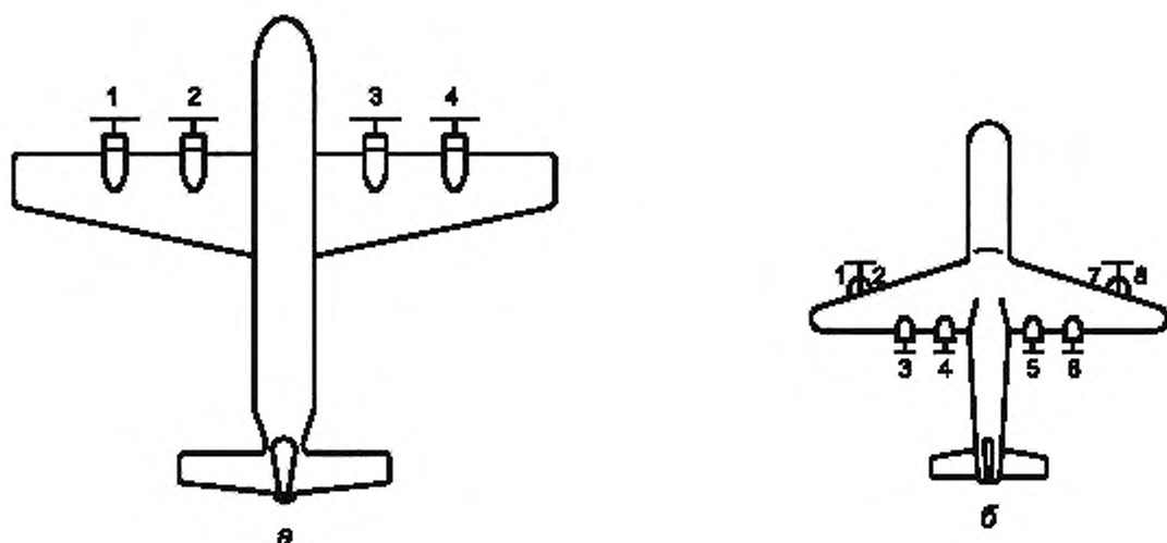
Рисунок 1 — Нумерация маршевых двигателей
