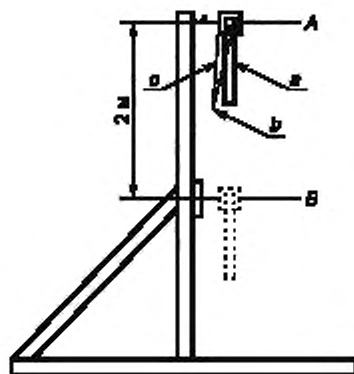
а — исходная длина провода, б — место соединения; с — удлинитель не более 2 м; А — начальное положение, в котором закрепляется измерительная аппаратура; В — конечное положение после окончания испытания измерительной аппаратуры
