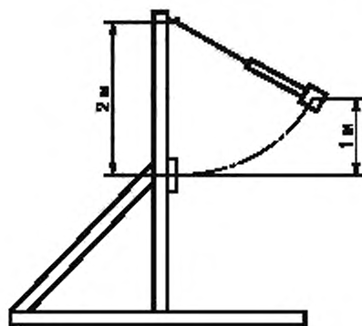
Рисунок А.1 — Испытание на механический удар
