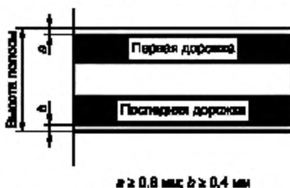
Рисунок 3 — Минимальная зона полосы
