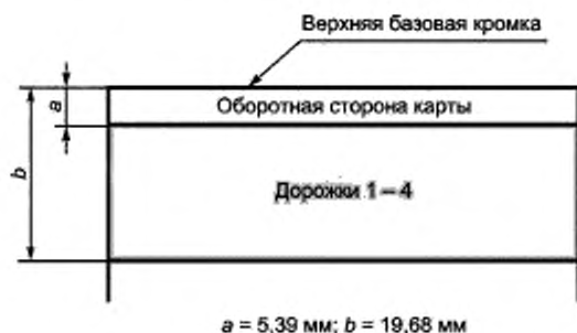
Рисунок 8 — Расположение и высота полосы при четырех дорожках
