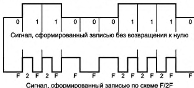
Рисунок В.1 — Кодирование F/2F
