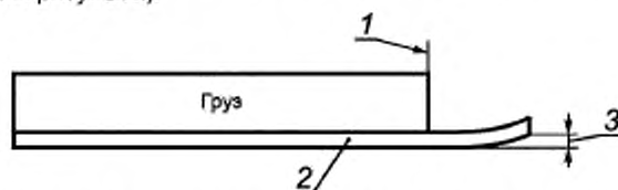
1 — нижний край магнитной полосы; 2 — испытываемая карта; 3 — загиб
