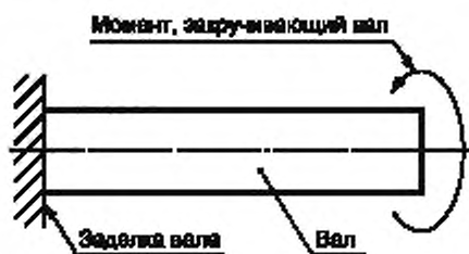
Рисунок 1 — Схема испытаний валов на прочность
