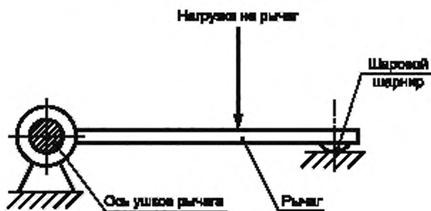
Рисунок 2 — Схема испытаний рычагов на прочность
