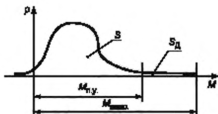
p — плотность распределения вероятности; M — момент на ступице колеса; S — общая площадь под кривой распределения в диапазоне M_{п.у.} \leq M \leq M_{макс.}
