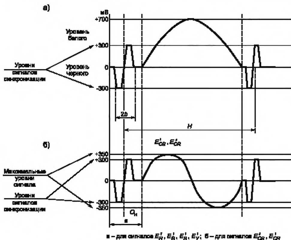
Рисунок 1 — Структура компонентных сигналов на интервале строки
