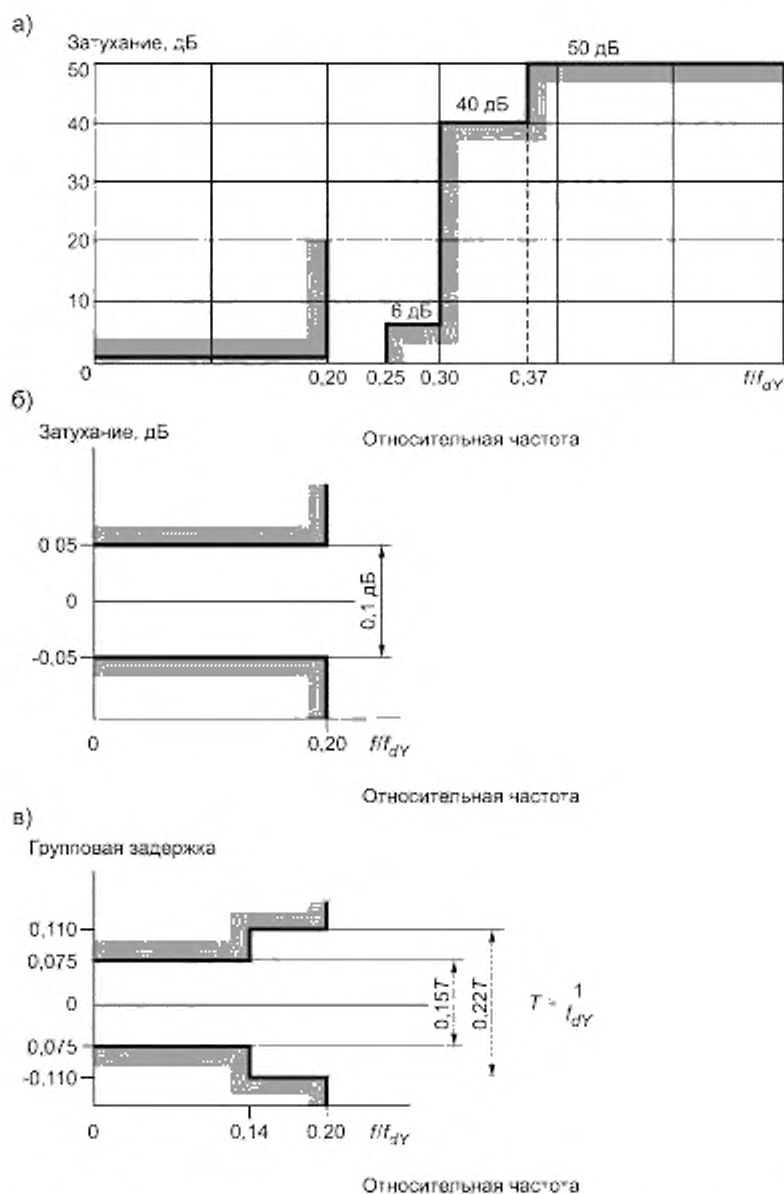
Рисунок 5 — Характеристики фильтров низких частот для сигналов E_{СВ} и E_{СВ}
