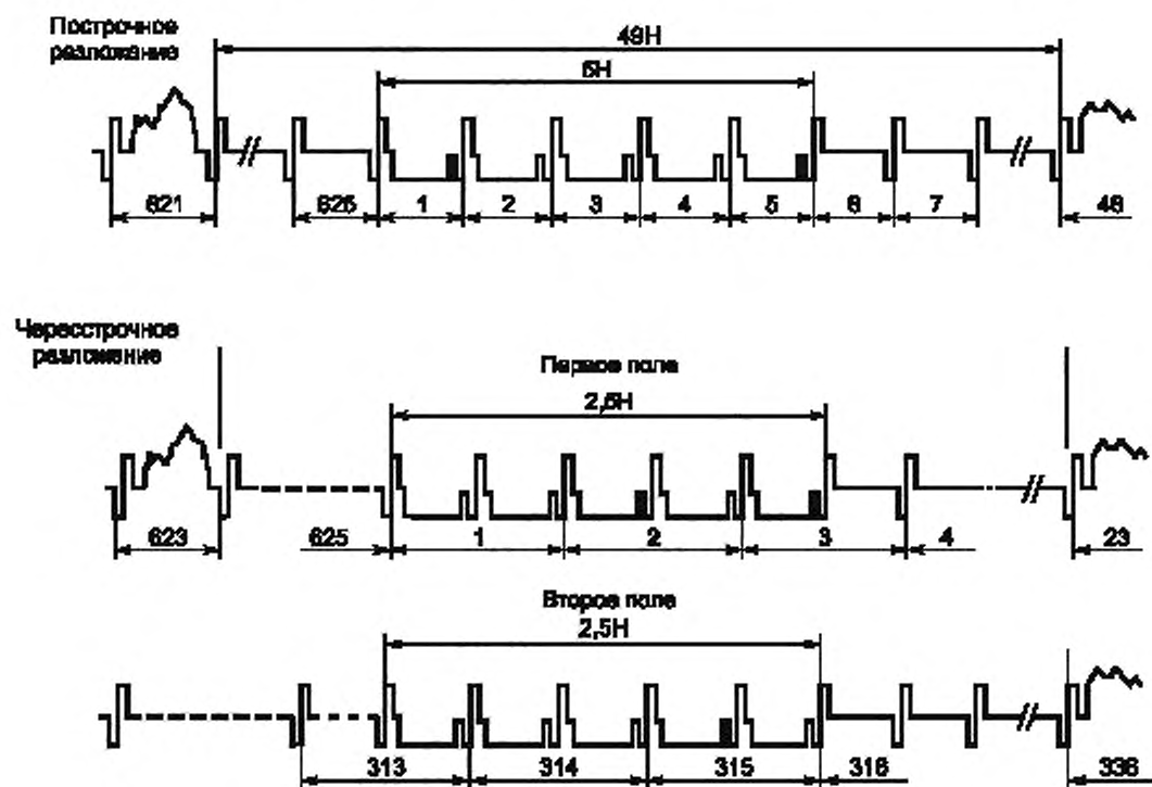
Рисунок 3 — Структура синхросигнала на интервале гашения поля
