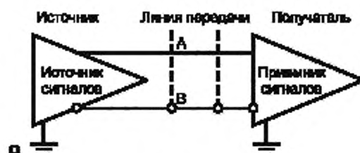
Рисунок 10 — Соединение источника сигналов и приемника сигналов
