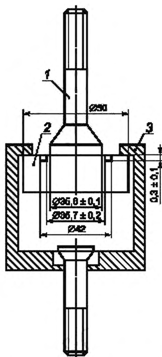
1 — испытательная головка; 2 — образец; 3 — захват
