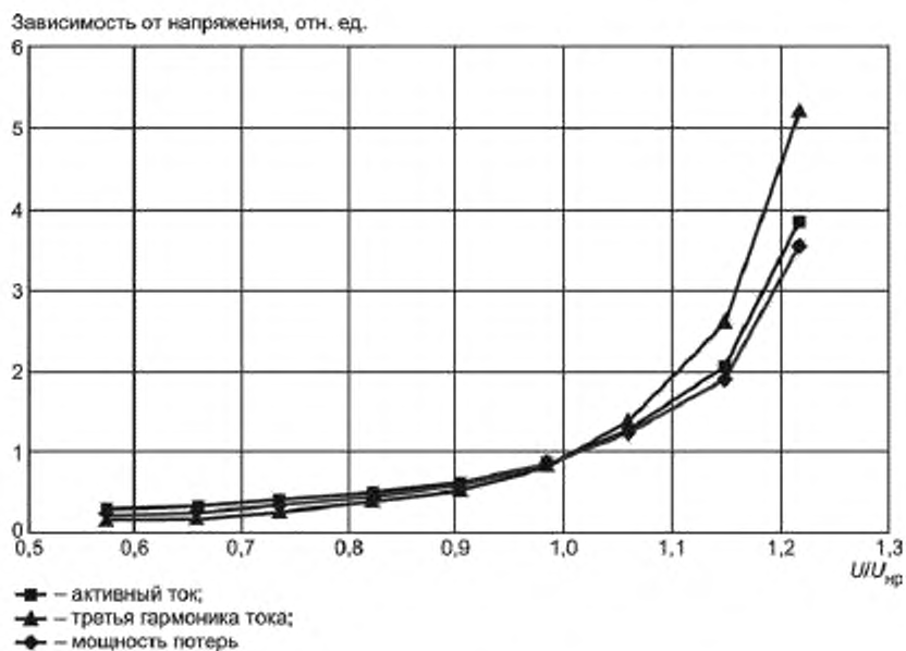
Рисунок 6 — Типичная нормализованная зависимость от напряжения при температуре +20 °С
