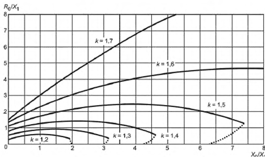
Рисунок А.2 — Соотношение между R_0 / X_1 и X_0 / X_1 для постоянных значений коэффициента замыкания на землю k , где R_1 = 0
