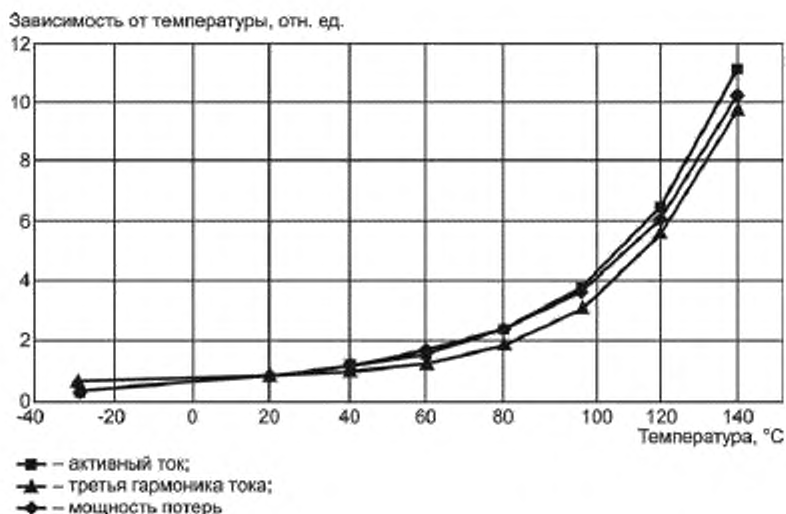
Рисунок 7 — Типичная нормализованная зависимость от температуры при наибольшем длительно допустимом рабочем напряжении U_{\text{пр}}
