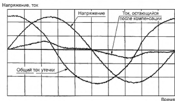
Рисунок 9 — Ток, остающийся после компенсации емкостного тока, при U_{np}
