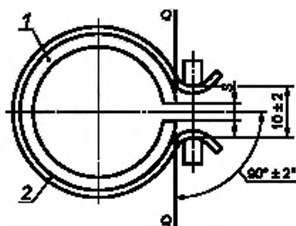
1— контролируемое кольцо; 2 — гибкая лента; S — зазор в замке кольца в рабочем состоянии
