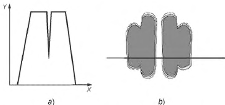
Рисунок В.1 — Профиль плотности пропускания расщепленной растровой точки на цветоделенной фотоформе (а) и изображение той же самой точки под микроскопом (b)
