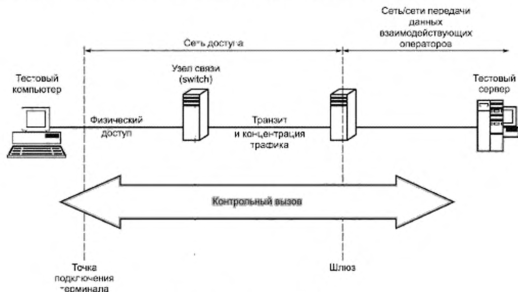
Рисунок Б.1 — Измерительная установка
