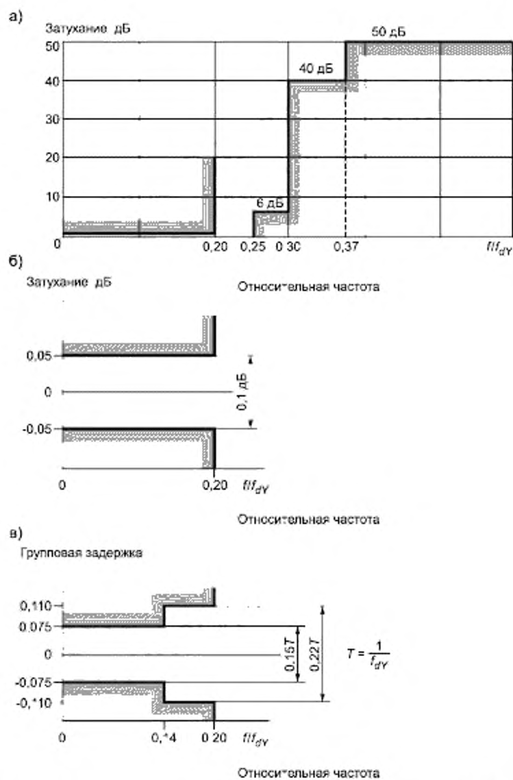
Рисунок А.2 — Характеристики фильтров низких частот для сигналов E_{сн}' и E_{св}'
