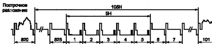
Рисунок 3 — Структура синхросигнала на интервале гашения поля
